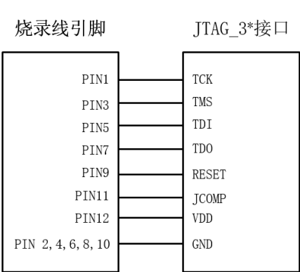
图7.9 烧录线与JTAG_3接口相连接
