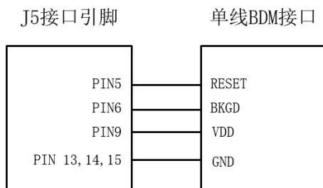
图7.14 J5接口与单线BDM接口相连接
