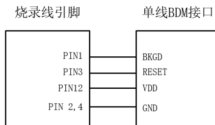
图7.15 烧录线与单线BDM接口相连接
