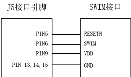
图7.22 J5接口与SWIM接口相连接
