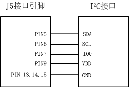
图7.26 J5接口与IIC接口相连接
