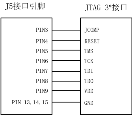
图7.8 J5接口与JTAG_3接口相连接
