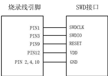
图7.11 烧录线与SWD接口相连接
