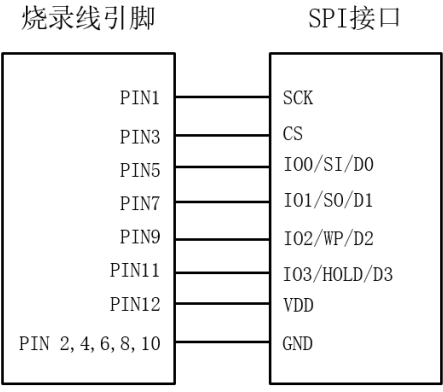
图7.19 烧录线与SPI接口相连接
