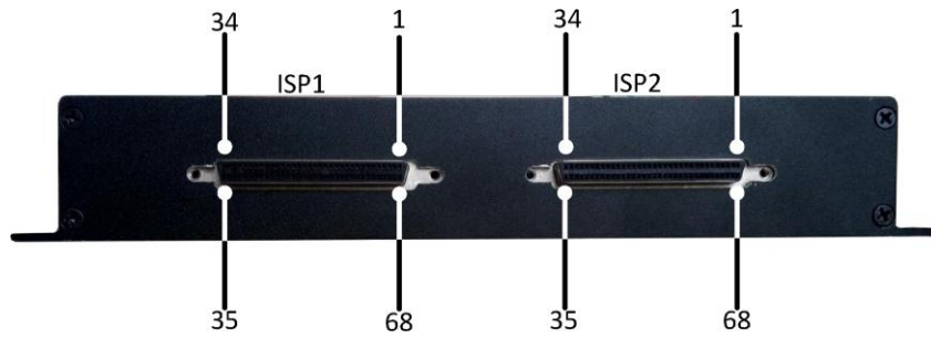
图3.2 烧录信号接口ISP1及ISP2
