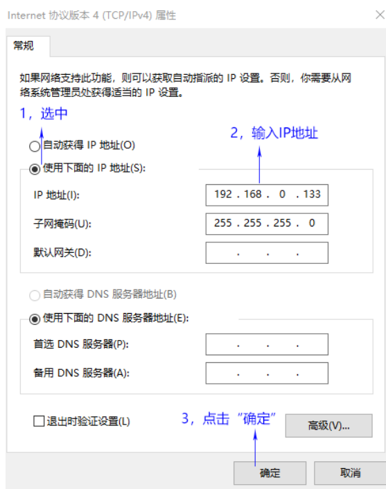
图4.7 修改计算机的IP地址，第4步
