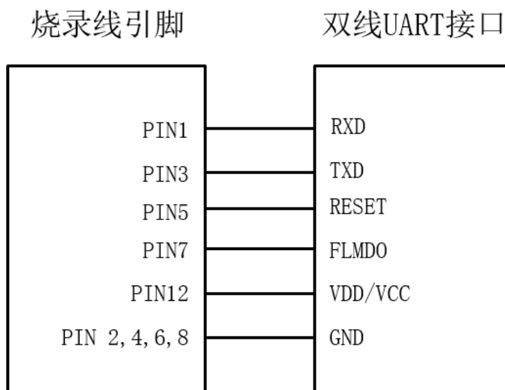
图7.9 S4/S8烧录线与双线UART接口相连接
