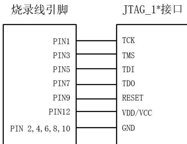
图7.3 S4/S8烧录线与JTAG_1接口相连接
