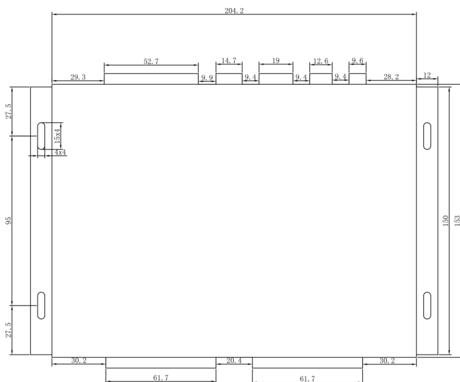
图3.4 烧录器俯视尺寸图（单位：mm）
