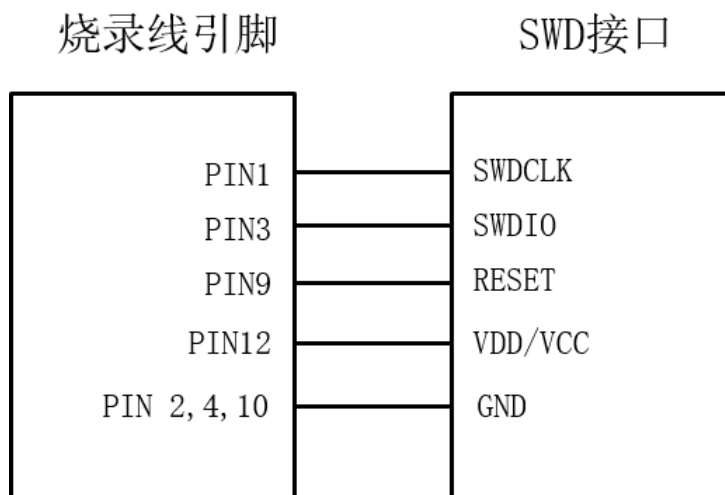
图7.13 S4/S8烧录线与SWD接口相连接
