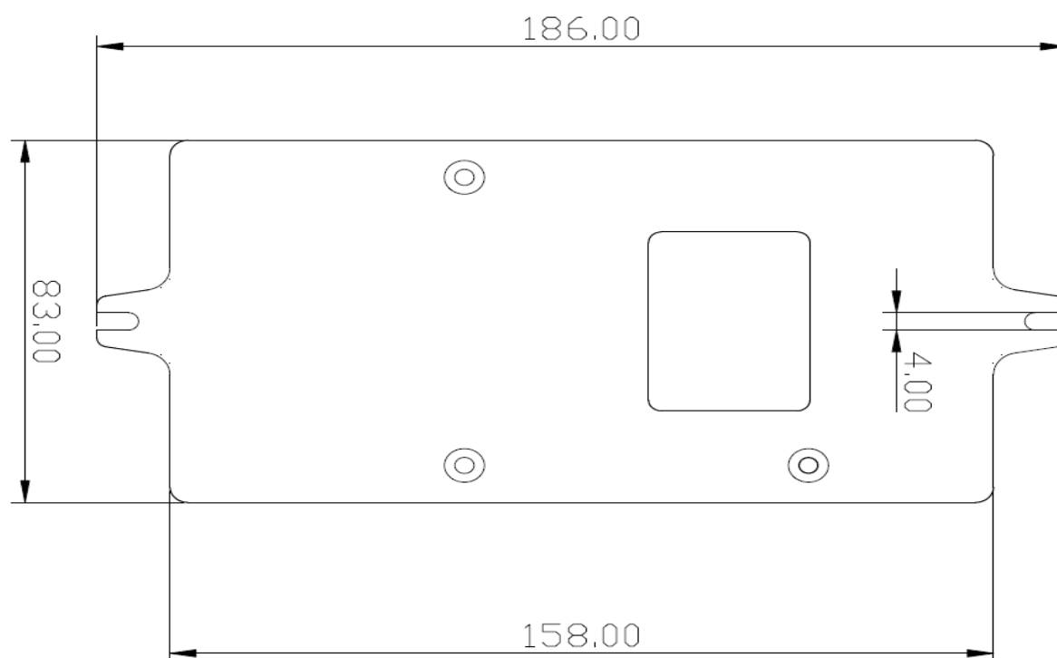
图 1-5 固定背板尺寸
