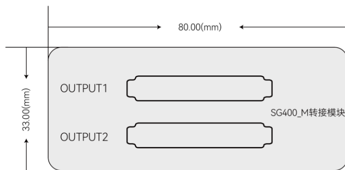
图 1-18SG400-M 转接模块尺寸
