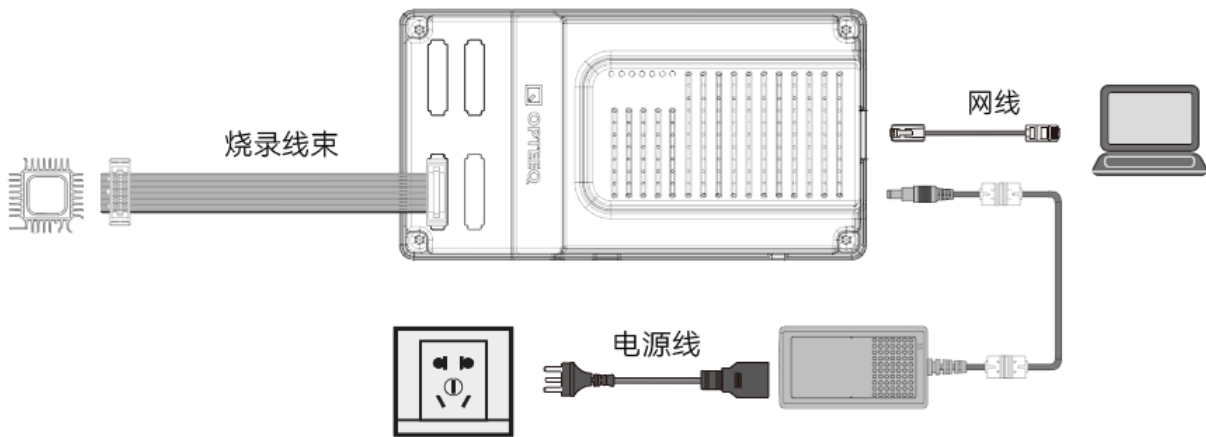
图 1-8SG400E 连接示意图
