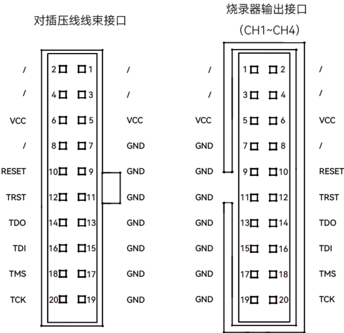
图 4-6 接口定义
