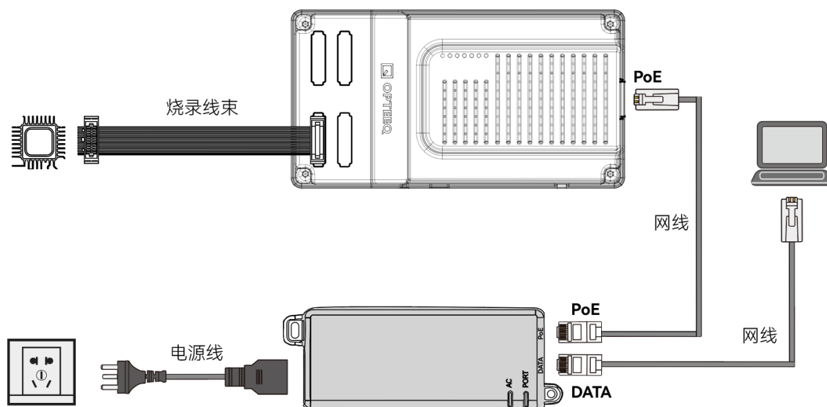
图 1-2SG400 连接示意图
