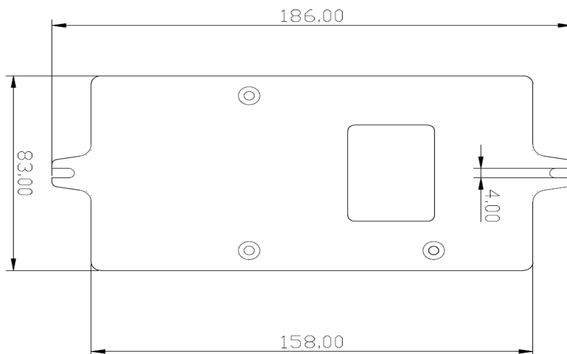
图 1-10 固定背板尺寸
