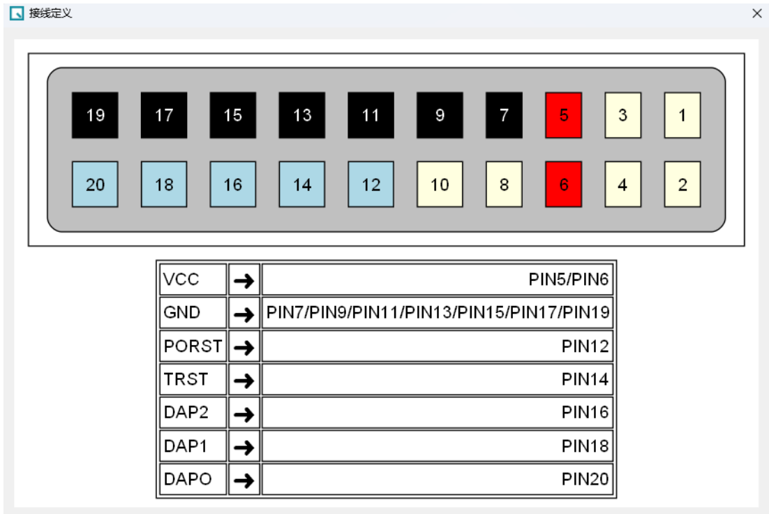
图 3-5 接线定义
