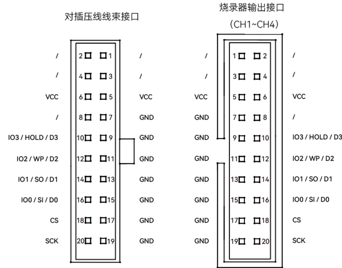
图 4-10 接口定义
