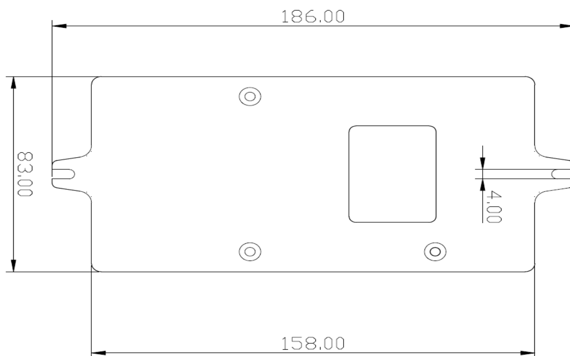
图 1-17 固定背板尺寸
