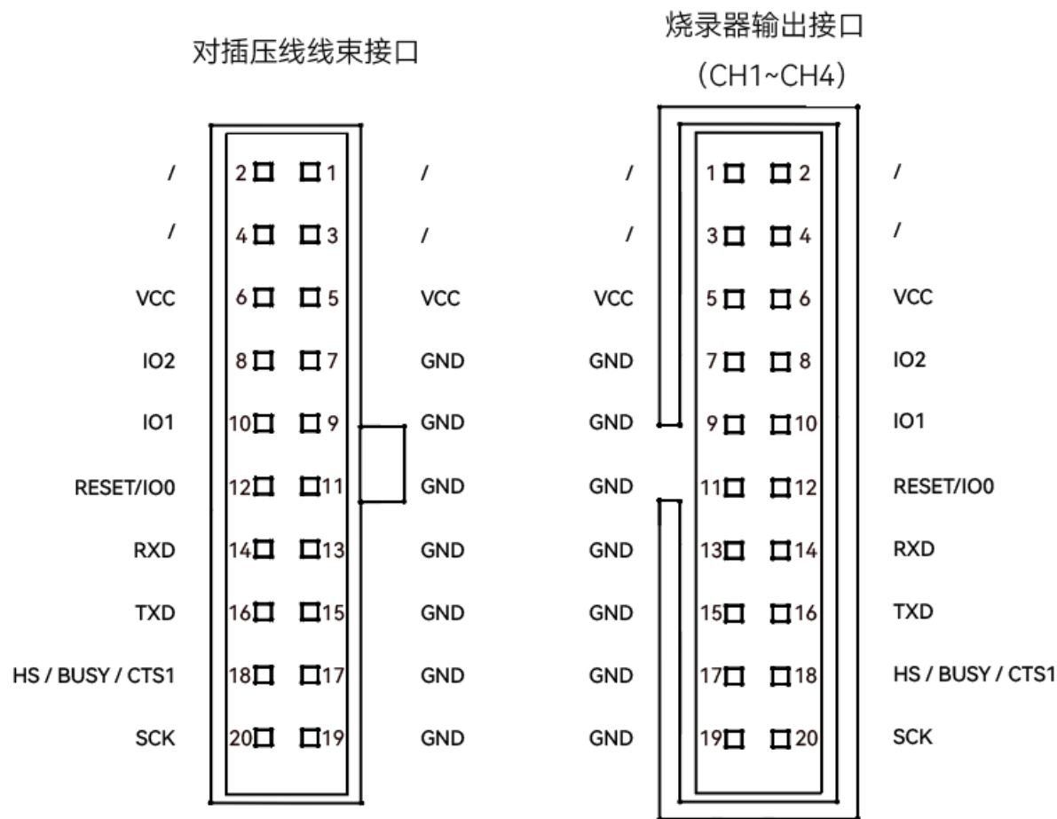
图 4-20 接口定义
