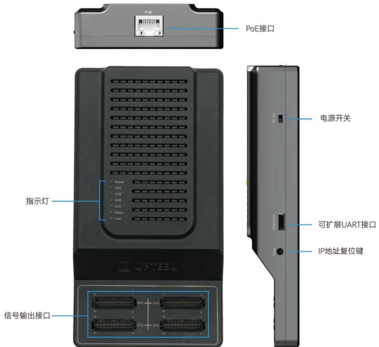
图 1-1SG400 外观及接口
