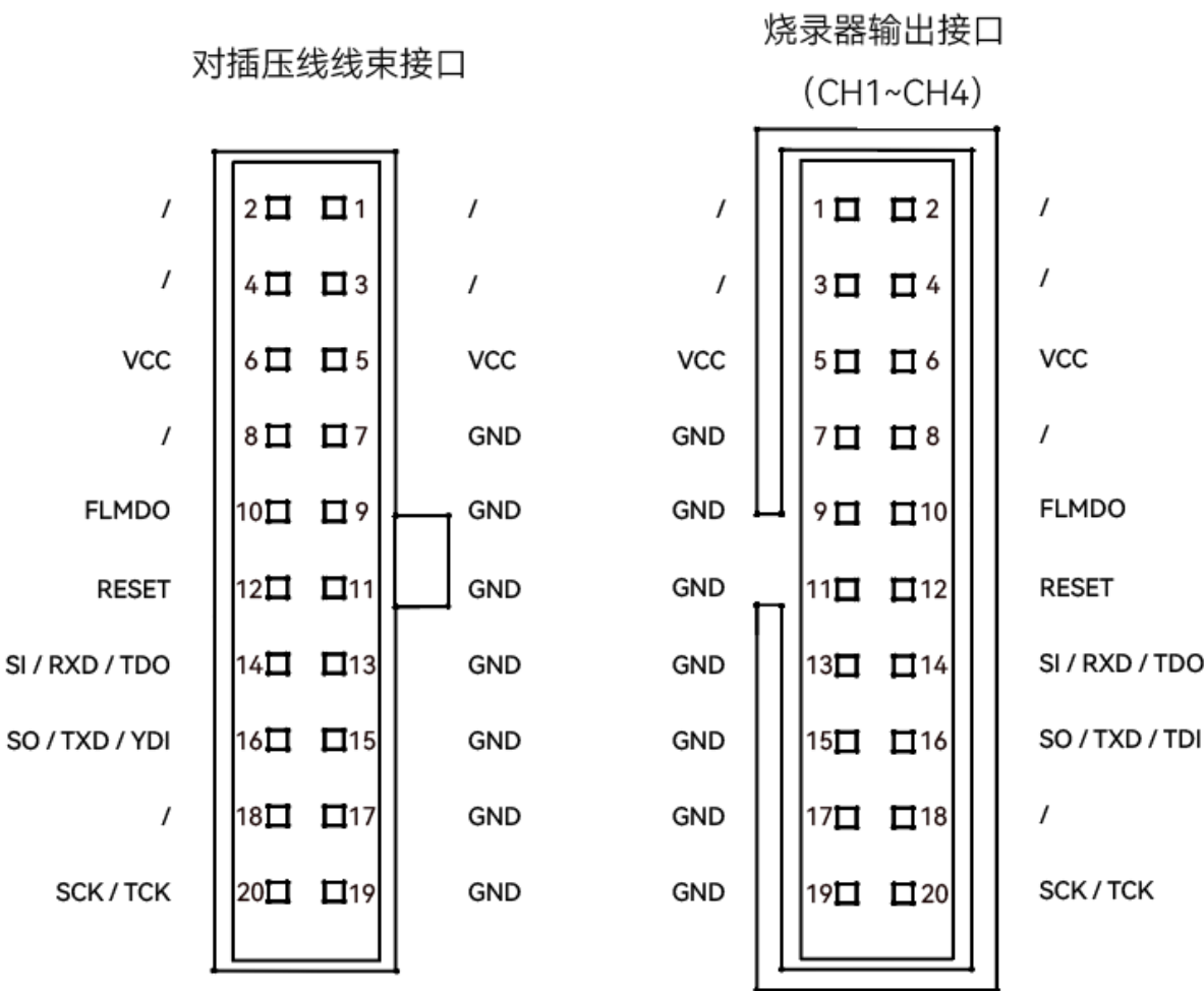
图 4-16 接口定义
