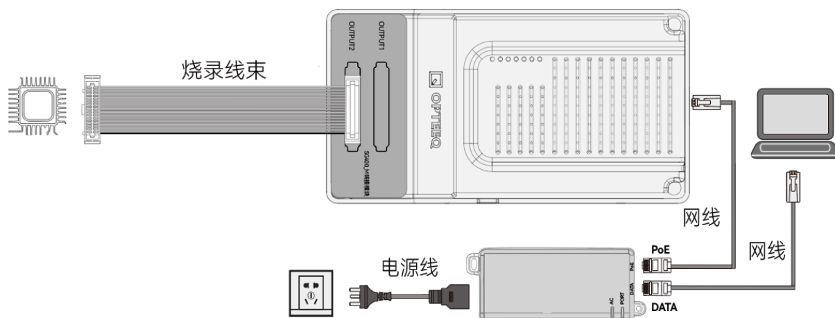
图 1-14SG400-M 连接示意图
