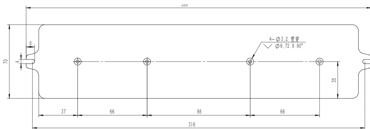
图 1-11 加长背板尺寸安装指南
