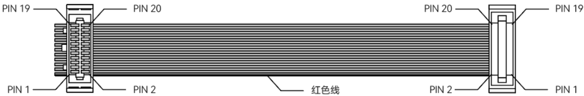
图 4-2 烧录线束示例图
