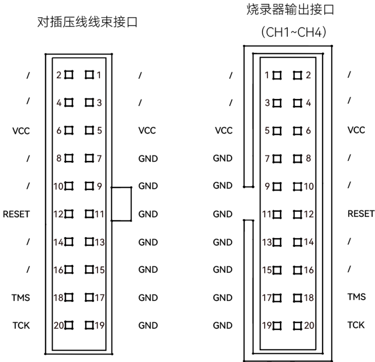
图 4-24 接口定义
