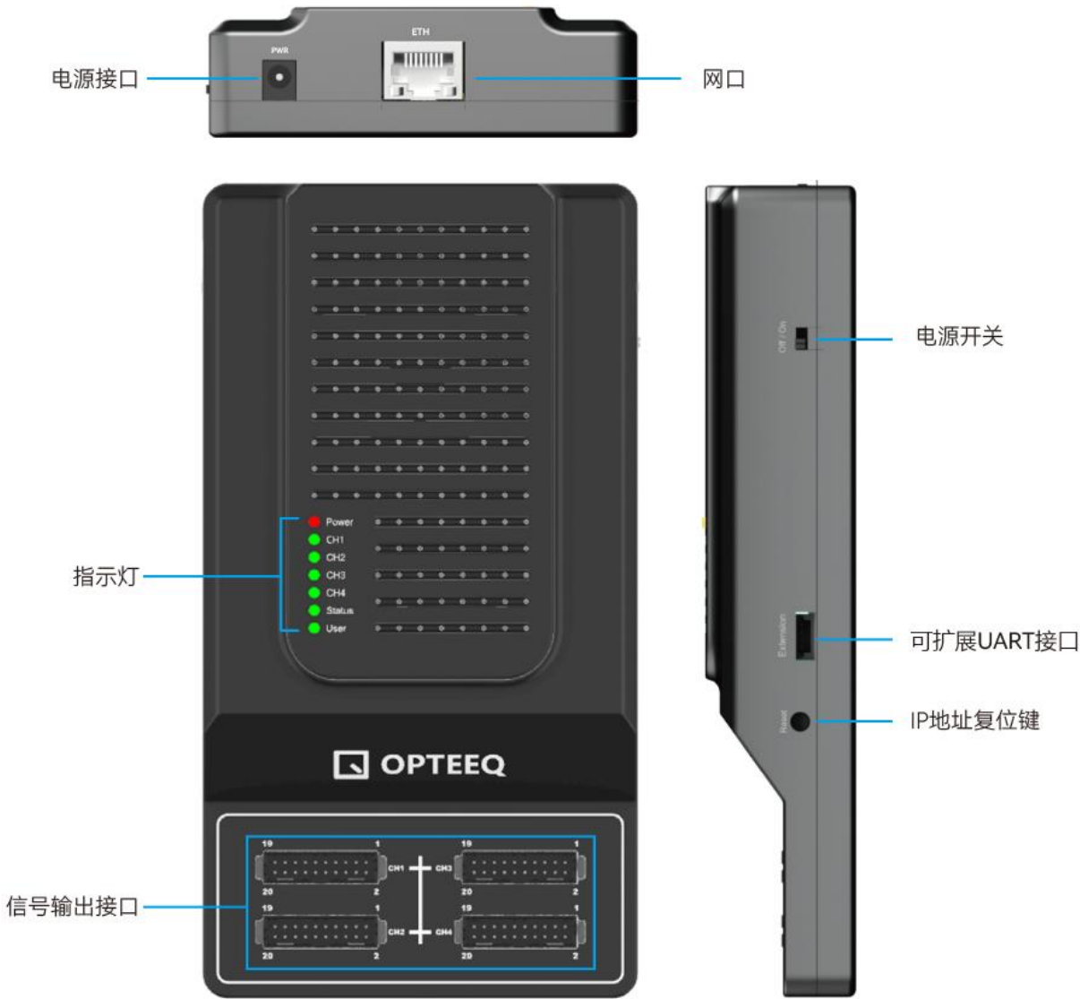
图 1-7SG400E 外观及接口
