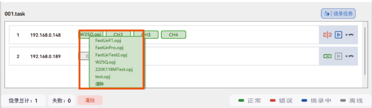
图 3-21 选择工程
