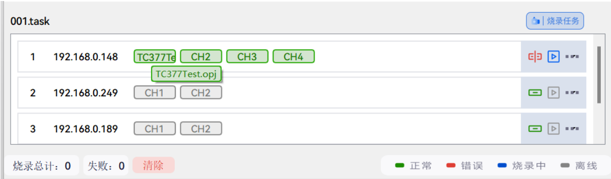
图 3-22 查看名称
