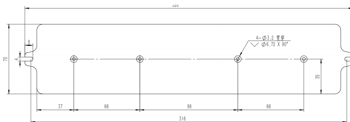
图 1-5 固定背板尺寸
