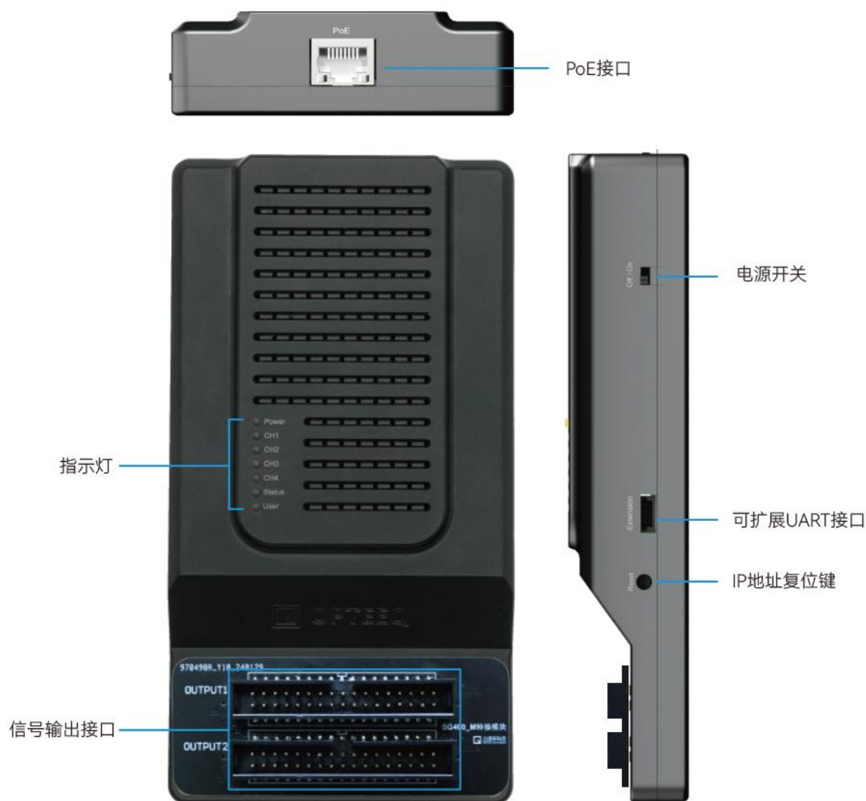
图 1-12SG400-M 外观及接口
