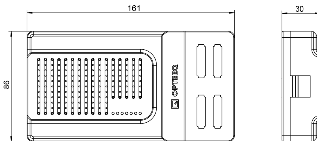
图 1-4 设备尺寸
