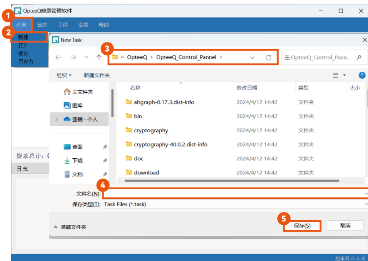
图 3-14 新建任务
