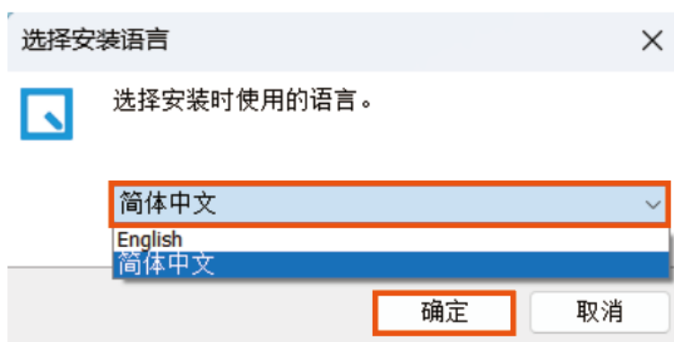
图 2-2 选择语言
