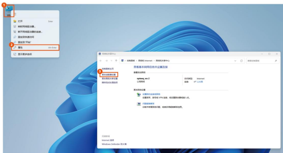
图 5-1 网络属性
