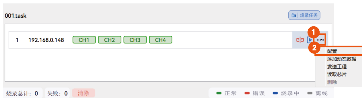
图 3-18 配置
