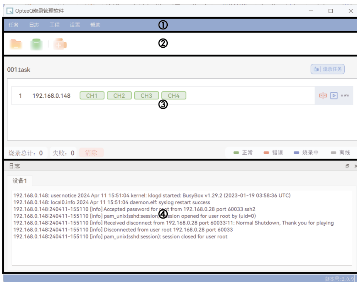
图 2-1 操作界面
