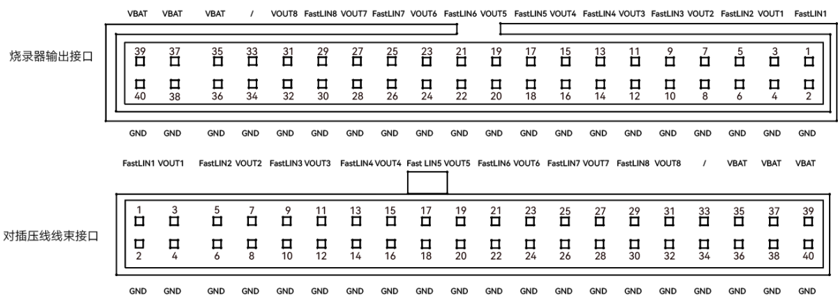
图 4-6 接口定义
