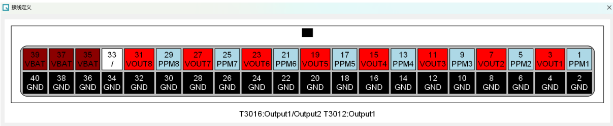
图 3-5 接线定义
