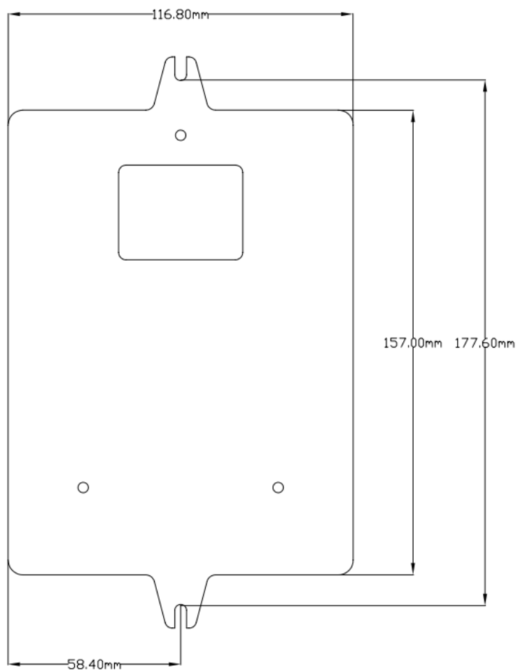
图 1-4 背板尺寸
