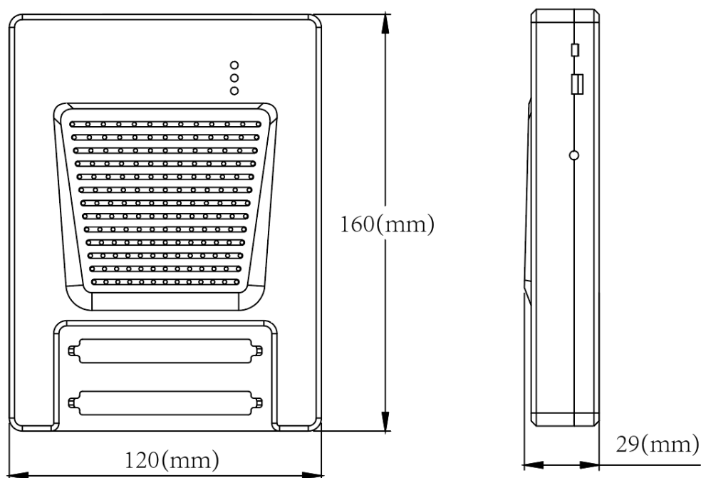
图 1-3 设备尺寸
