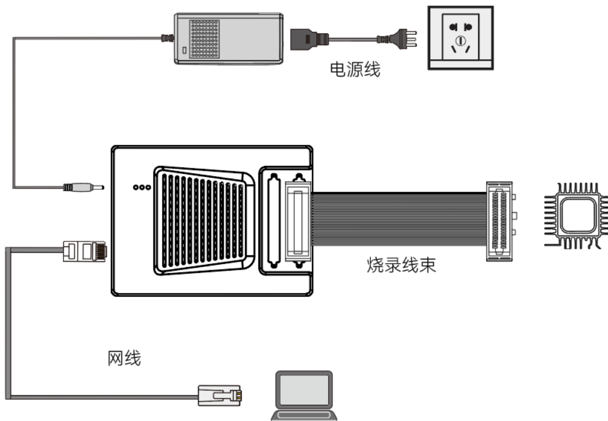
图 2-1 连接示意图
