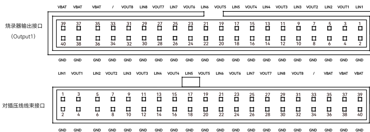
图 4-1 Output1 接口定义
