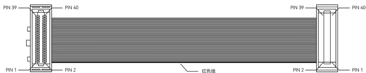
图 4-3 烧录线束示例图
