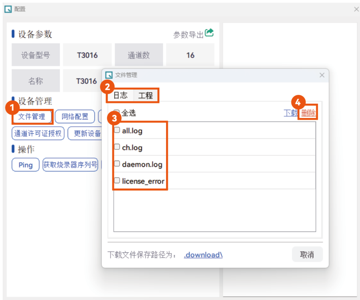
图 3-44 删除文件
