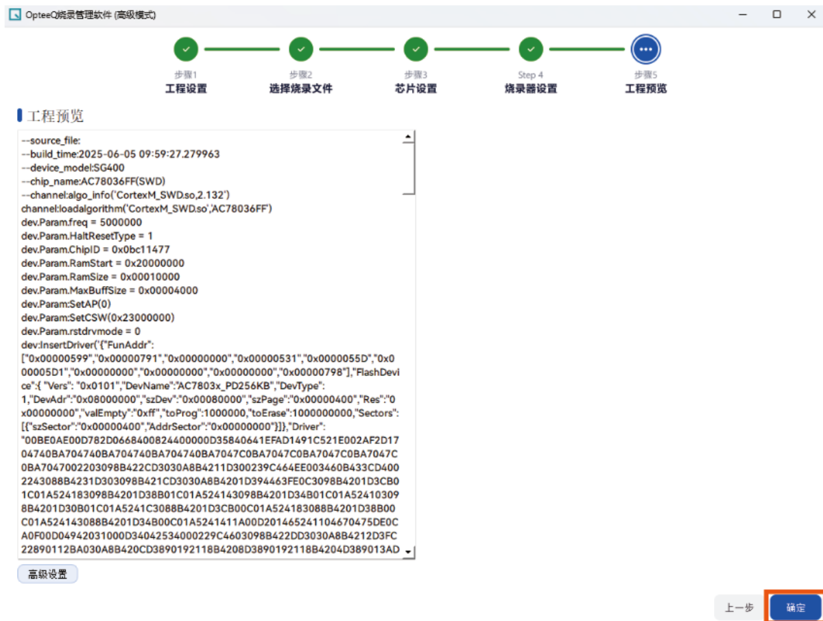
图 3-10 工程预览
