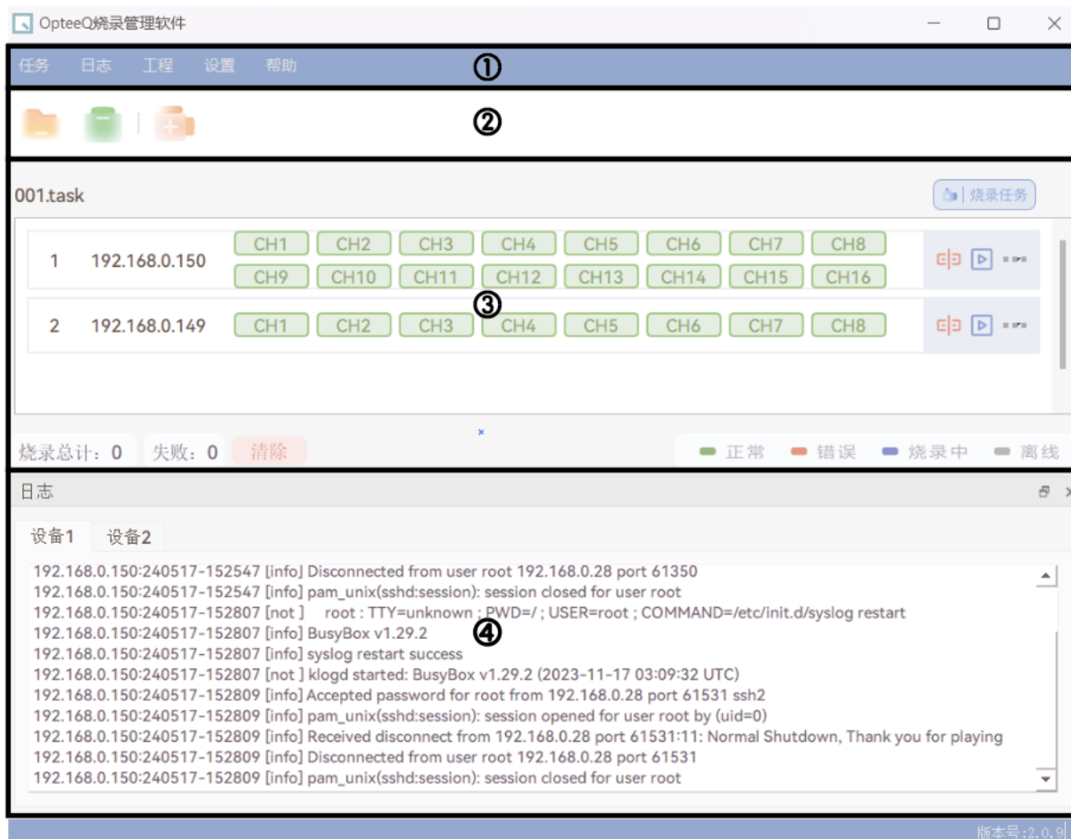
图 1-2 操作界面
