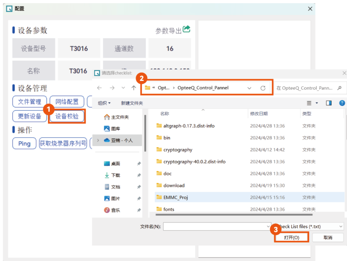
图 3-54 设备校验
