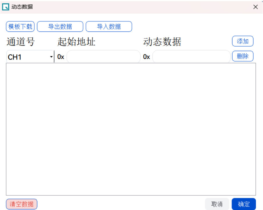
图 3-22 动态数据
