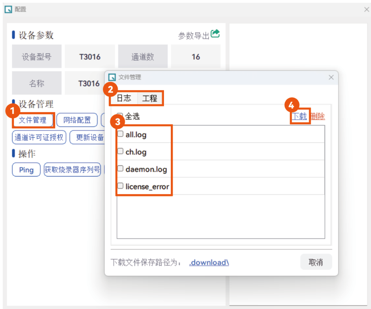
图 3-43 下载文件
