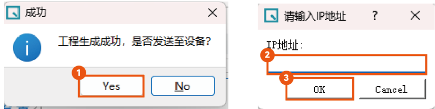
图 3-12 发送工程
