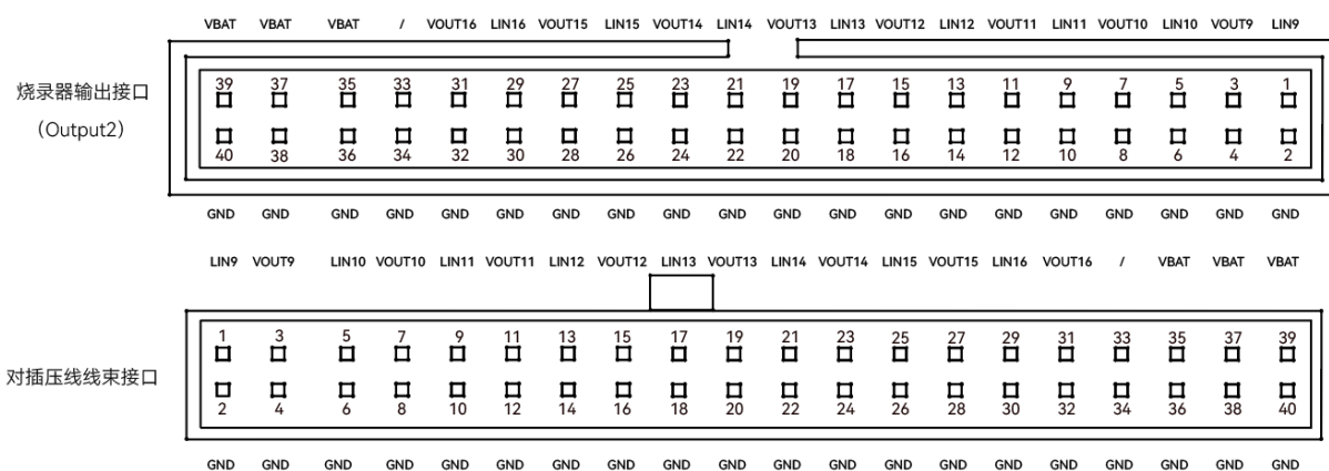
图 4-2 Output2 接口定义
