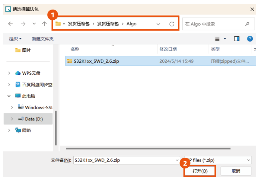
图 3-35 选择文件
