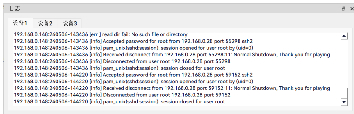
图 3-63 日志区
