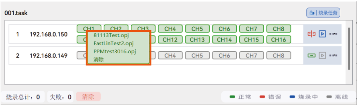
图 3-20 选择工程
