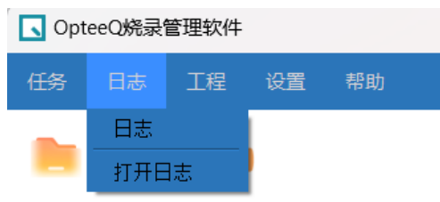
图 3-61 日志菜单
