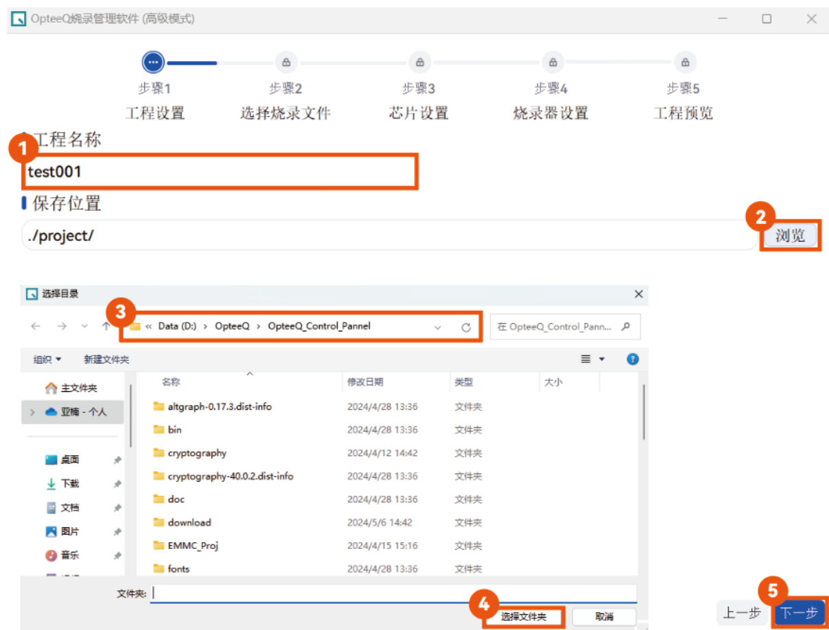
图 3-6 工程设置
