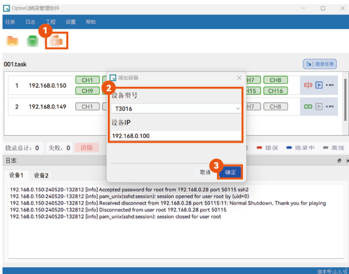
图 3-14 添加设备
